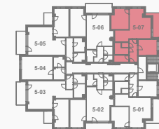
PŮDORYS
